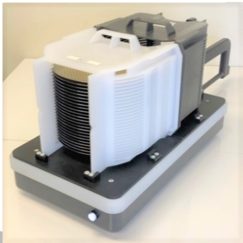
AHWT - 自動ウエハ移載機
